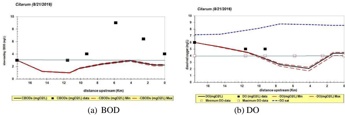
Gambar 5. (a) Profil BOD dan (b) DO setelah dilakukan pengurangan beban pencemar
