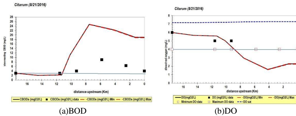
Gambar 6. (a) Profil BOD dan (b) DO pada kondisi debit maksimum
