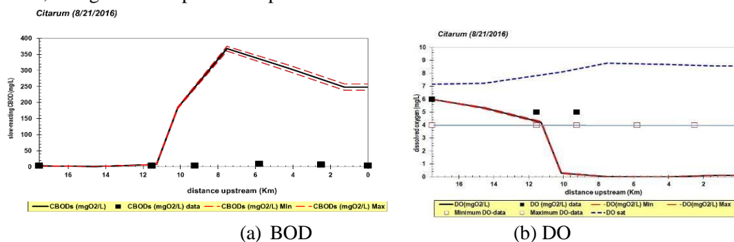
Gambar 4. (a) Profil BOD dan (b) DO pada kondisi debit minimum
