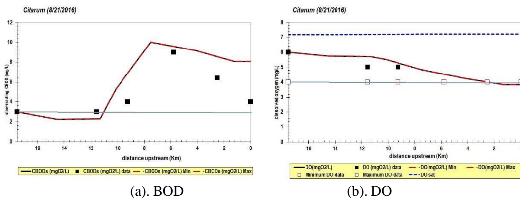
Gambar 2. (a) Profil BOD dan (b) DO pada kondisi eksisting
