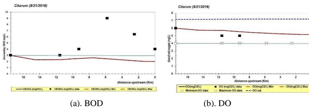
Gambar 3. Grafik (a) BOD dan (b) DO dibandingkan baku mutu, setelah dilakukan pengurangan beban pencemaran
