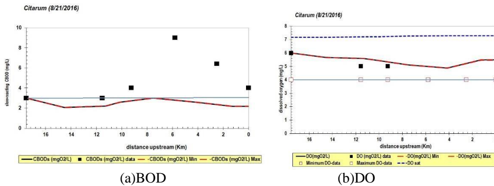
Gambar 7. Profil (a)BOD dan (b)DO setelah dilakukan pengurangan beban pencemaran
